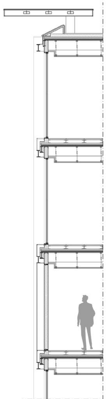
sezione A:A
